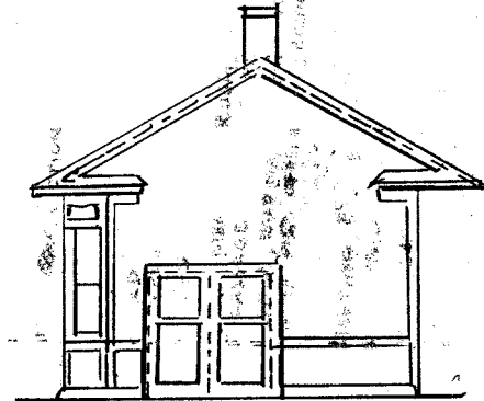
END ELEVATION
